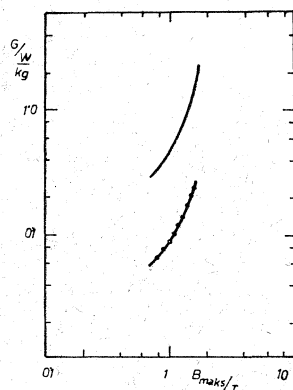
Sl. 4. Usporedba gubitaka u jezgri ( G ) za konvencionalnu Fe_{82}B_{10}Si_8 slitinu (puna linija), amorfnu slitinu Fe_{82}B_{10}Si_8 (kružići) iste debljine pri sinusnoj indukciji magnetskog polja B frekvencije 60 Hz
