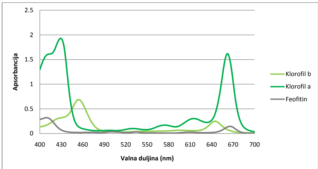
Slika 18. Apsorpcijski spektri klorofila a i b i feofitina (otopljenih u acetonu) u vidljivom dijelu spektra (400 – 700 nm).
