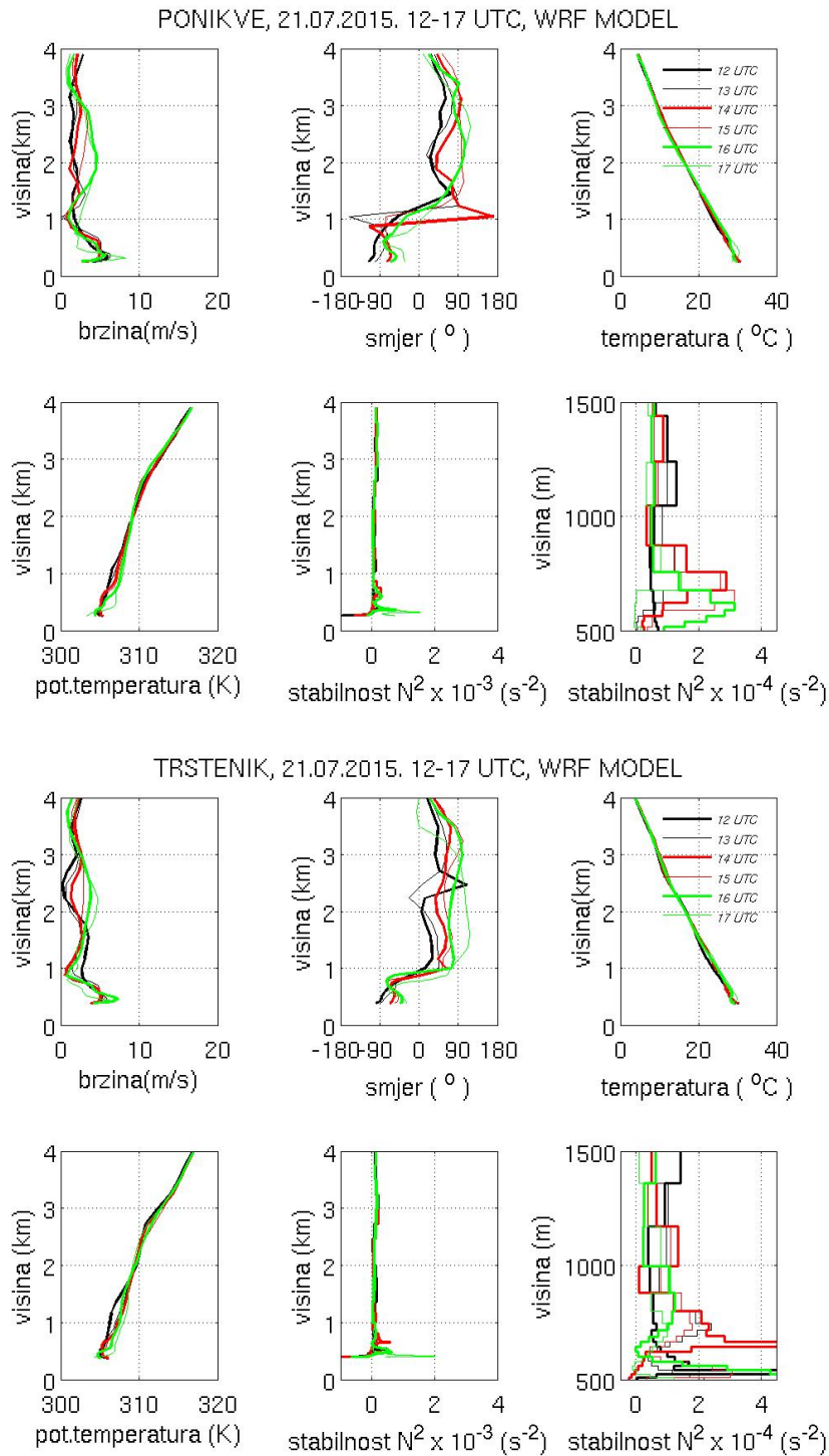
Slika 6.9: Vertikalni profili brzine vjetrova (gore lijevo), smjera vjetrova (gore sredina), temperature zraka (gore desno), potencijalne temperature (dolje lijevo), kvadrata uzgonske frekvencije (dolje sredina) i uvećani profil kvadrata uzgonske frekvencije (dolje desno) za Ponikve (slika gore) i Trstenik (slika dolje) 21.7.2015. od 12 do 17 UTC dobiveni modelom WRF.
