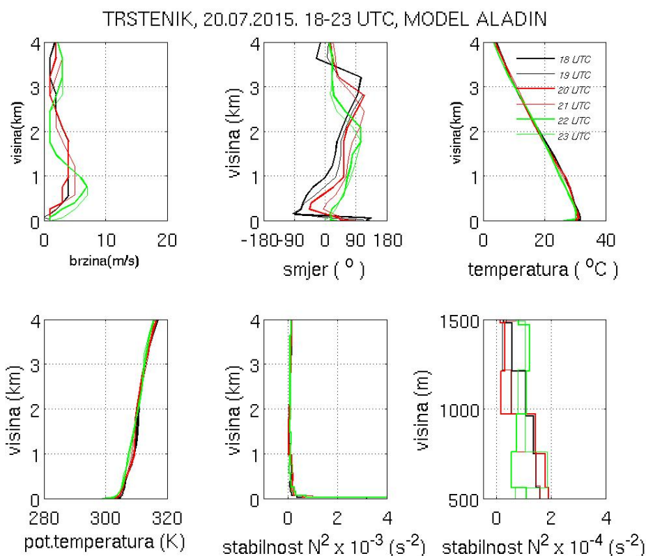
Slika 4.27: Vertikalni profili brzine vjetrova (gore lijevo), smjera vjetrova (gore sredina), temperature zraka (gore desno), potencijalne temperature (dolje lijevo), kvadrata uzgonske frekvencije (dolje sredina) i uvećani profil kvadrata uzgonske frekvencije (dolje desno) za Ponikve (slika gore) i Trstenik (slika dolje) 20.7.2015. od 18 do 23 UTC dobiveni modelom ALADIN/HR.
