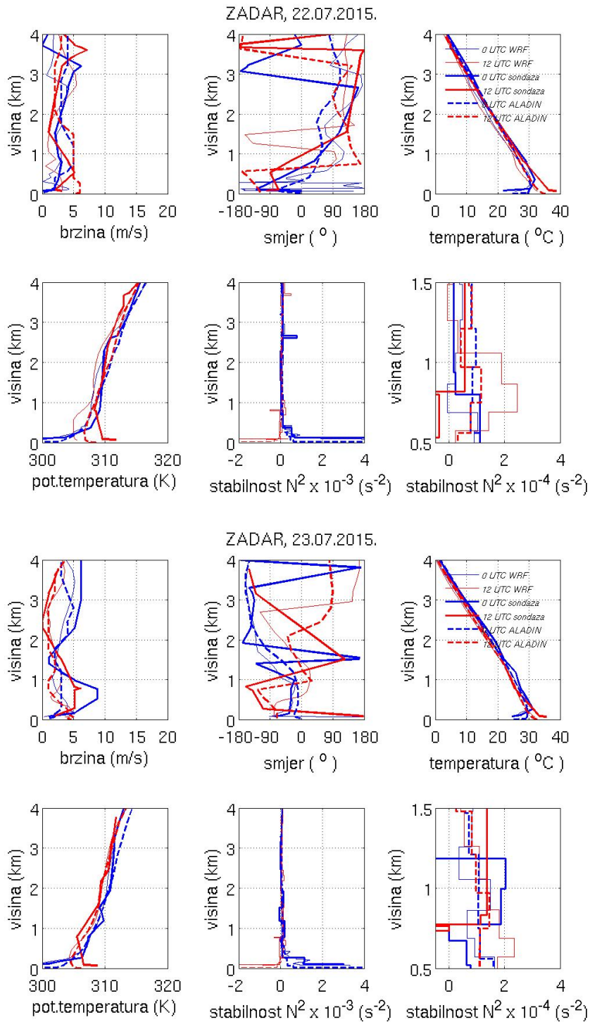
Slika 6.6: Vertikalni profili brzine vjeta (gore lijevo), smjera vjeta (gore sredina), temperature zraka (gore desno), potencijalne temperature (dolje lijevo), kvadrata uzgonske frekvencije (dolje sredina) i uvećani profil kvadrata uzgonske frekvencije (dolje desno) za Zadar 22.7.2015. u 00 i 12 UTC (gore) i 23.7.2015. u 00 i 12 UTC (dolje) . Mjerenja su prikazana debljom linijom, model WRF tanjom, a model ALADIN/HR debljom iscrtkanom.
