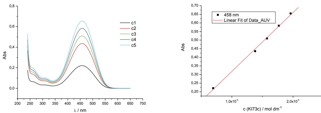
Slika D 2. lijevo: UV/Vis spektar spoja KI73C u koncentracijskom rasponu 6,95 \times 10^{-6} - 1,96 \times 10^{-5} \text{ mol dm}^{-3} pri pH 5,00, u kakovilnatnom puferu c = 0,05 \text{ mol dm}^{-3} ; desno: ovisnost apsorbancije spoja KI73C o koncentraciji pri 458 nm
