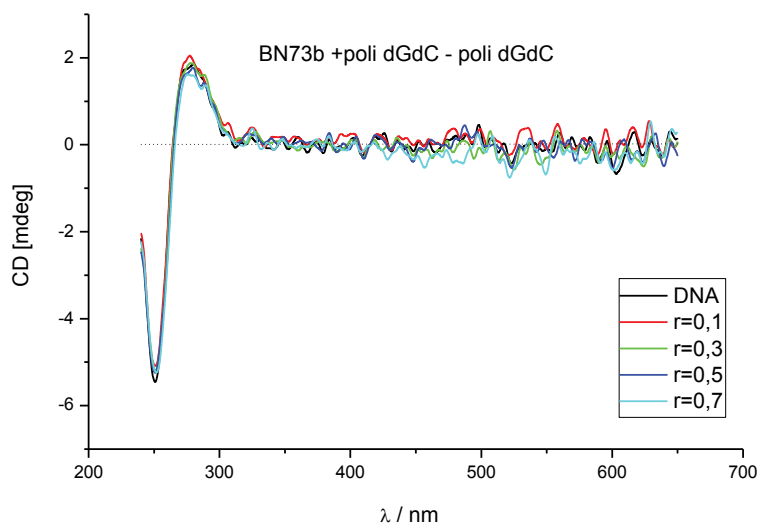
Slika 38. CD titracija poli dGdC – poli dGdC ( c = 2 \times 10^{-5} \text{ mol dm}^{-3} ) sa spojem BN73B, različitim molarnim omjerima r = [\text{spoj}] / [\text{polinukleotid}] ( \text{pH} = 7,08 , Na – kakodilatni pufer, I = 0,05 \text{ mol dm}^{-3} )
