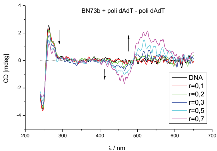
Slika 37. CD titracija poli dAdT – poli dAdT ( c = 2 \times 10^{-5} \text{ mol dm}^{-3} ) sa spojem BN73B, različitim molarnim omjerima r = [\text{spoj}] / [\text{polinukleotid}] ( \text{pH} = 7,08 , Na – kakodilatni pufer, I = 0,05 \text{ mol dm}^{-3} )
