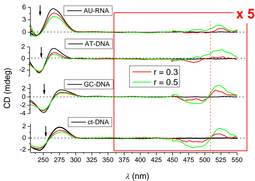
Slika 10. CD titracija dvolančane DNA i dvolančane RNA ( \blacksquare ; c = 2 \times 10^{-5} \text{ mol dm}^{-3} ) s spojem 2 u molarnim omjerima r_{[\text{spoj 2}]/[\text{polinukleotid}]} = 0,3 ( \blacksquare ) i 0,5 ( \blacksquare ). Potrebno je zamjetiti kako je okvirom označeni raspon 450-550 nm pomnožen s 5 za bolju vidljivost. Provedeno pri pH 7 uz natrijev kakodilatni pufer, I = 0,05 \text{ mol dm}^{-3} .
