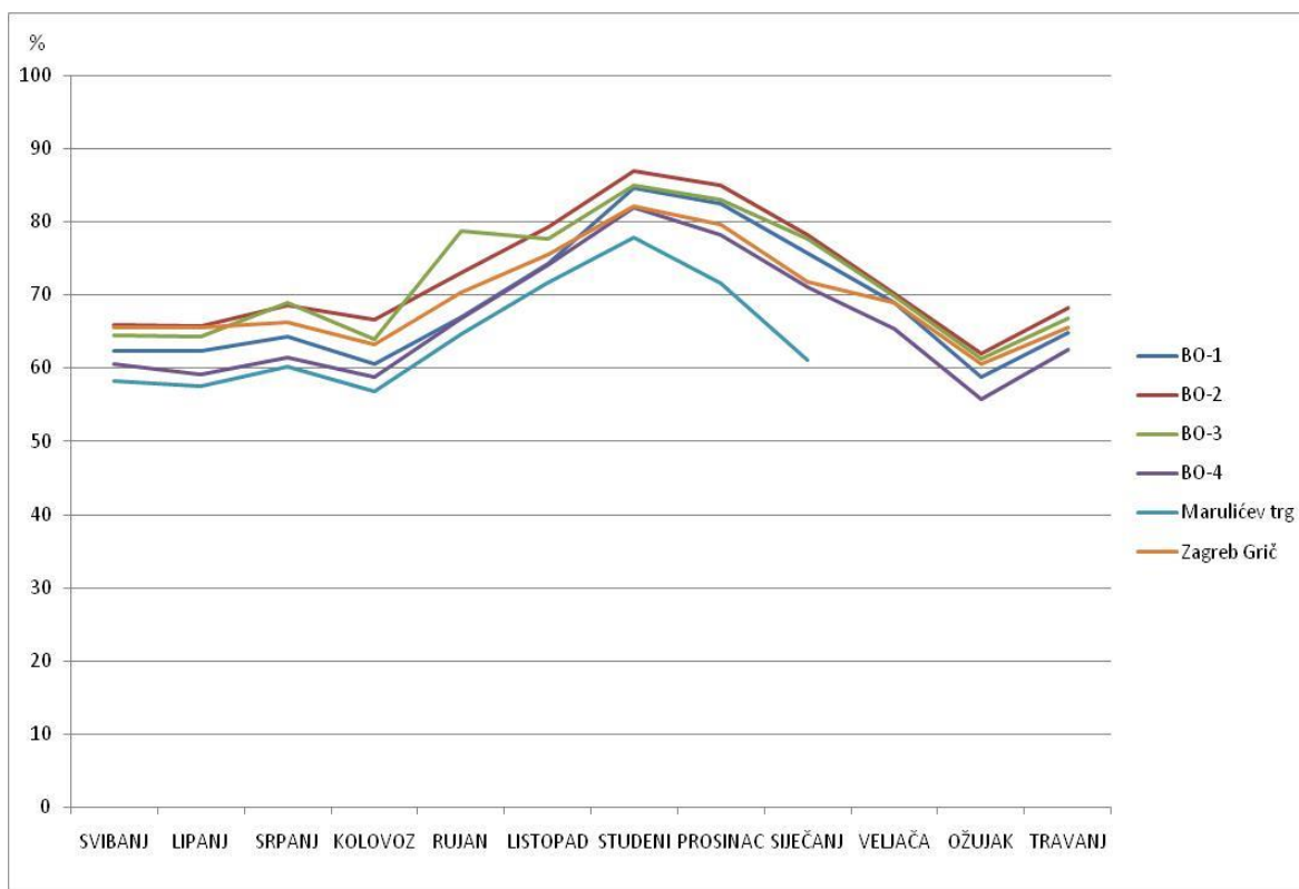
Sl. 12. Mjesečne vrijednosti relativne vlažnosti zraka analiziranih mjernih postaja za razdoblje od 1.5.2018. do 30.4.2019. godine
