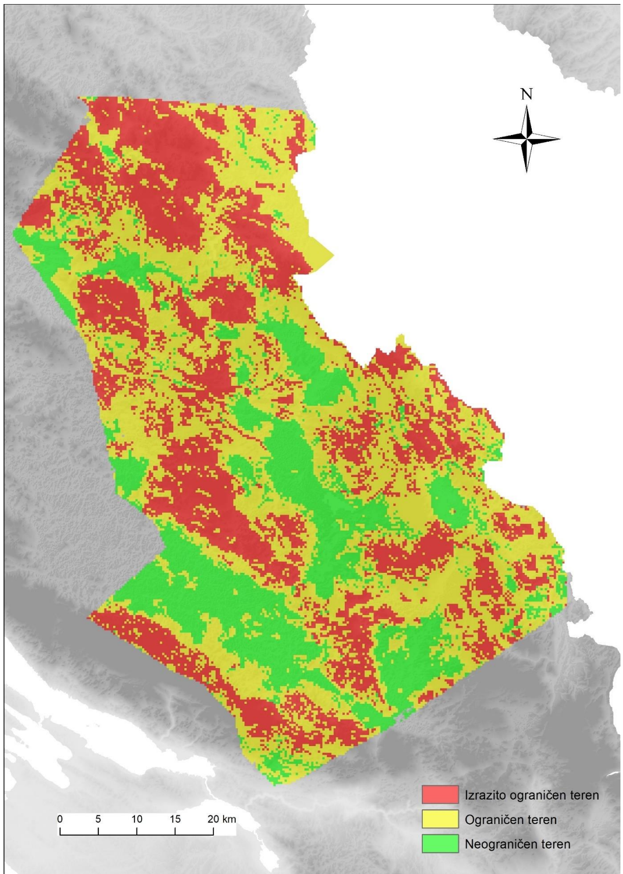
Slika 18: Prohodnost terena
