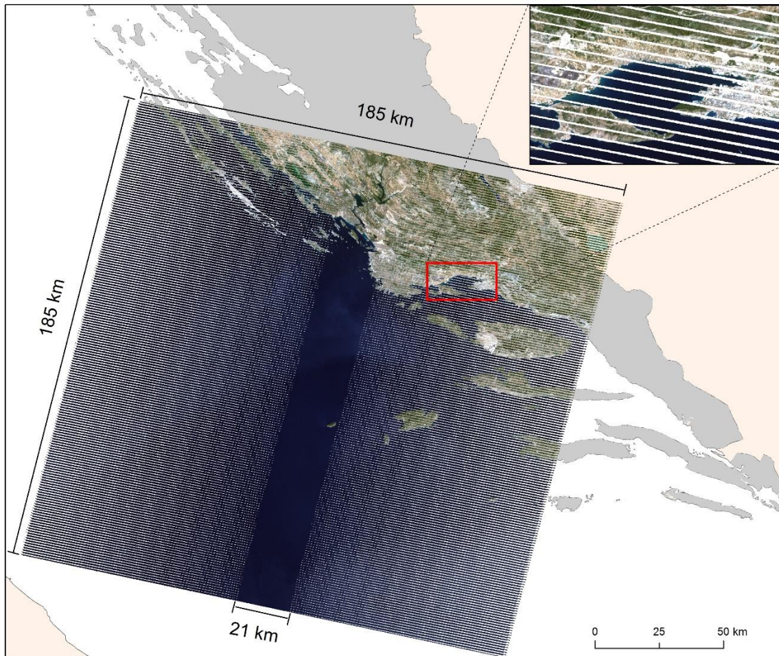
Sl. 7. Scena ETM+ senzora nakon kvara scan line corrector instrumenta Landsat 7 ETM+, 19.8.2012., RGB kompozicija: 3 2 1
