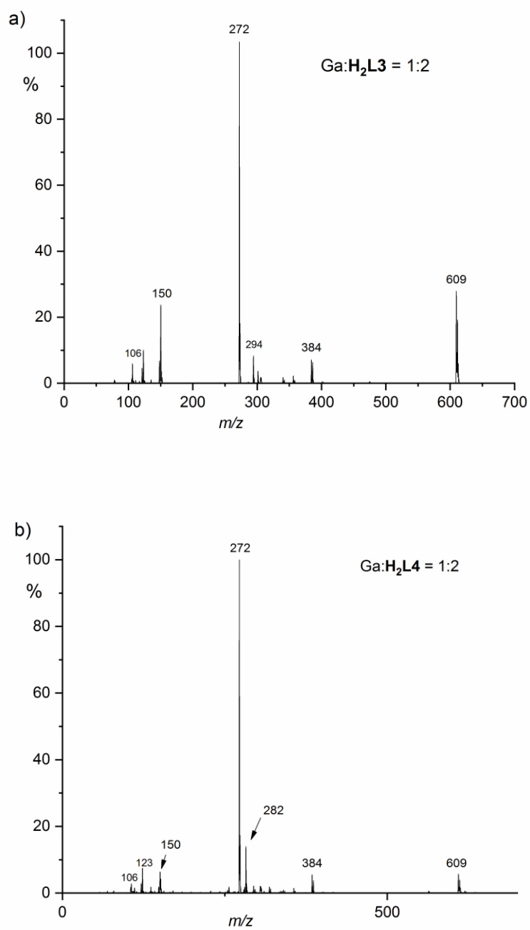
Slika D7. MS spektar otopine izoliranih kompleksa Ga 3+ sa H 2 L 3 (a) i H 2 L 4 (b)
