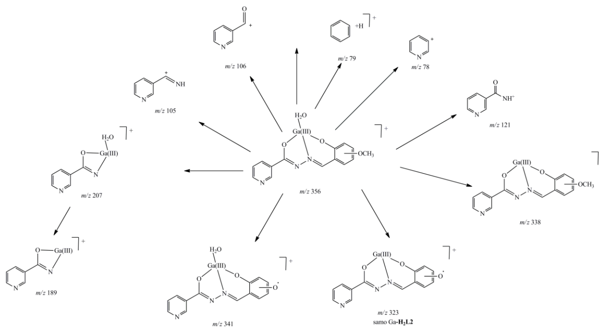
Slika 4.13. Predložena shema fragmentacije ionskog kompleksa [Ga(L)(H_2O)]^+ m/z 356 uz kolizijsku energiju od 30 V
