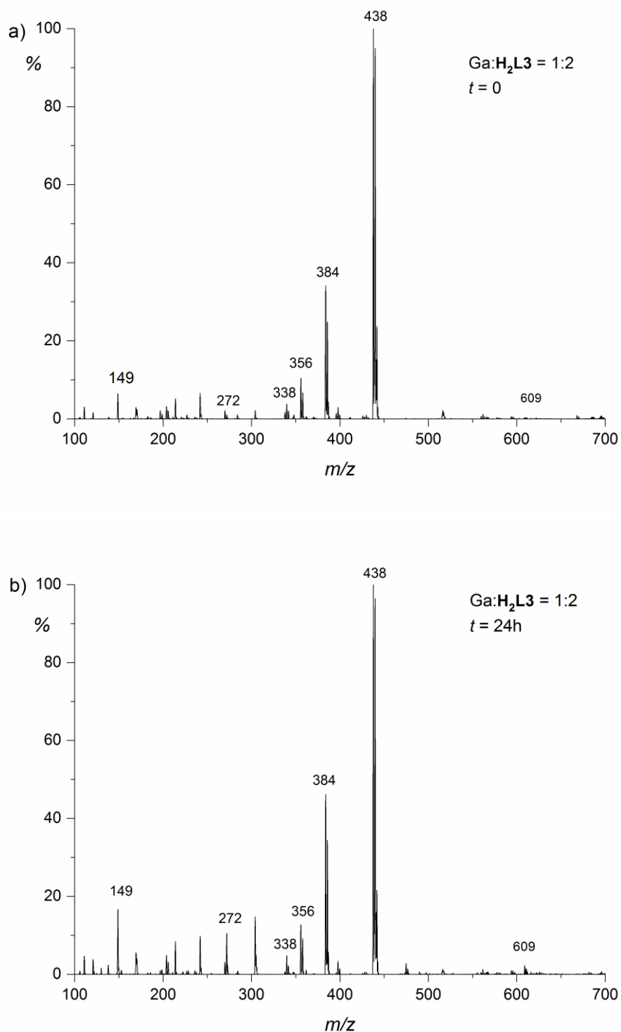
Slika 4.3. Spektri masa otopine galijeva(III) perklorata i hidrazona \text{H}_2\text{L3} i u omjeru 1:2 ( c(\text{H}_2\text{L3}) = 5 \times 10^{-4} \text{ mol L}^{-1} , c(\text{Ga}^{3+}) = 2,5 \times 10^{-4} \text{ mol L}^{-1} ) u sustavu metanol/voda 1/1 uz perklornu kiselinu ( c(\text{HClO}_4) = 0,003 \text{ mol L}^{-1} ; pH = 2,52), a) odmah po priprevi otopine i b) 24 sata nakon priprave otopine. Napon fragmentora 135 V.
