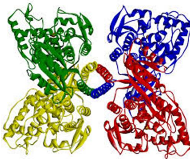
Slika 10. Nativna struktura PAH (kod sisavaca) [7]
