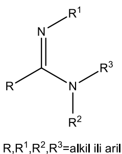
Slika 12. Općenita strukturna formula amidina
