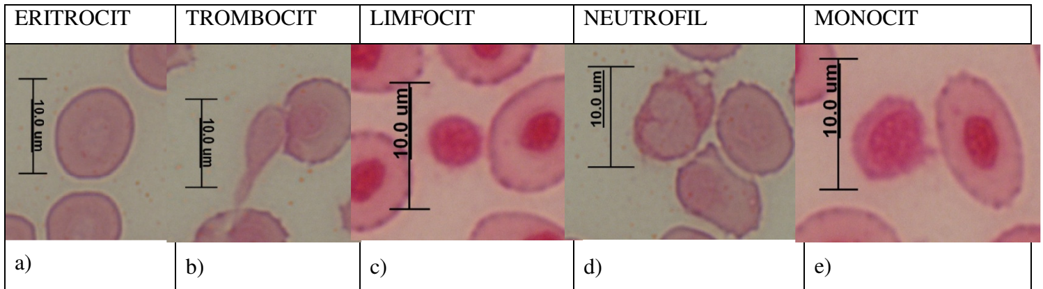
Slika 20. Rezultati reakcije ANBE. Pozitivne reakcije smo dobili kod limfocita c), slabu reakciju kod neutrofila d) i monocita e). Eritrociti a) i trombociti b) nisu pokazali pozitivno obojenje.
