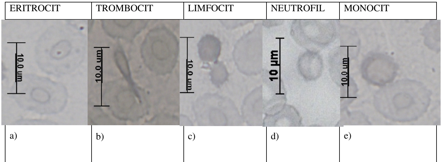
Slika 18. Rezultati bojanja tehnikom SB. Jezgre svih stanica su nebojane. Eritrociti a) ne pokazuju reakciju kao ni trombociti b), dok se kod limfocita c), neutrofila d) i monocita e) vide reakcije u citoplazmi kao tamnije obojano područje.
