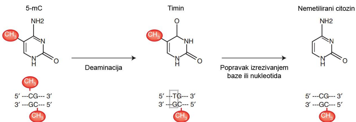
Slika 2 – Primjer demetilacije 5-metilcotozina, 5-mC. Deaminacijom se 5-mC konvertira u uracil kojeg enzimi popravka DNA izrezivanjem baze ili nukleotida zamjenjuju citozinom. Signal za popravak je pogrešno sparena baza u molekuli DNA: T/G umjesto C/G. Slika je preuzeta i prilagođena iz rada Day i Sweatt (2010).
