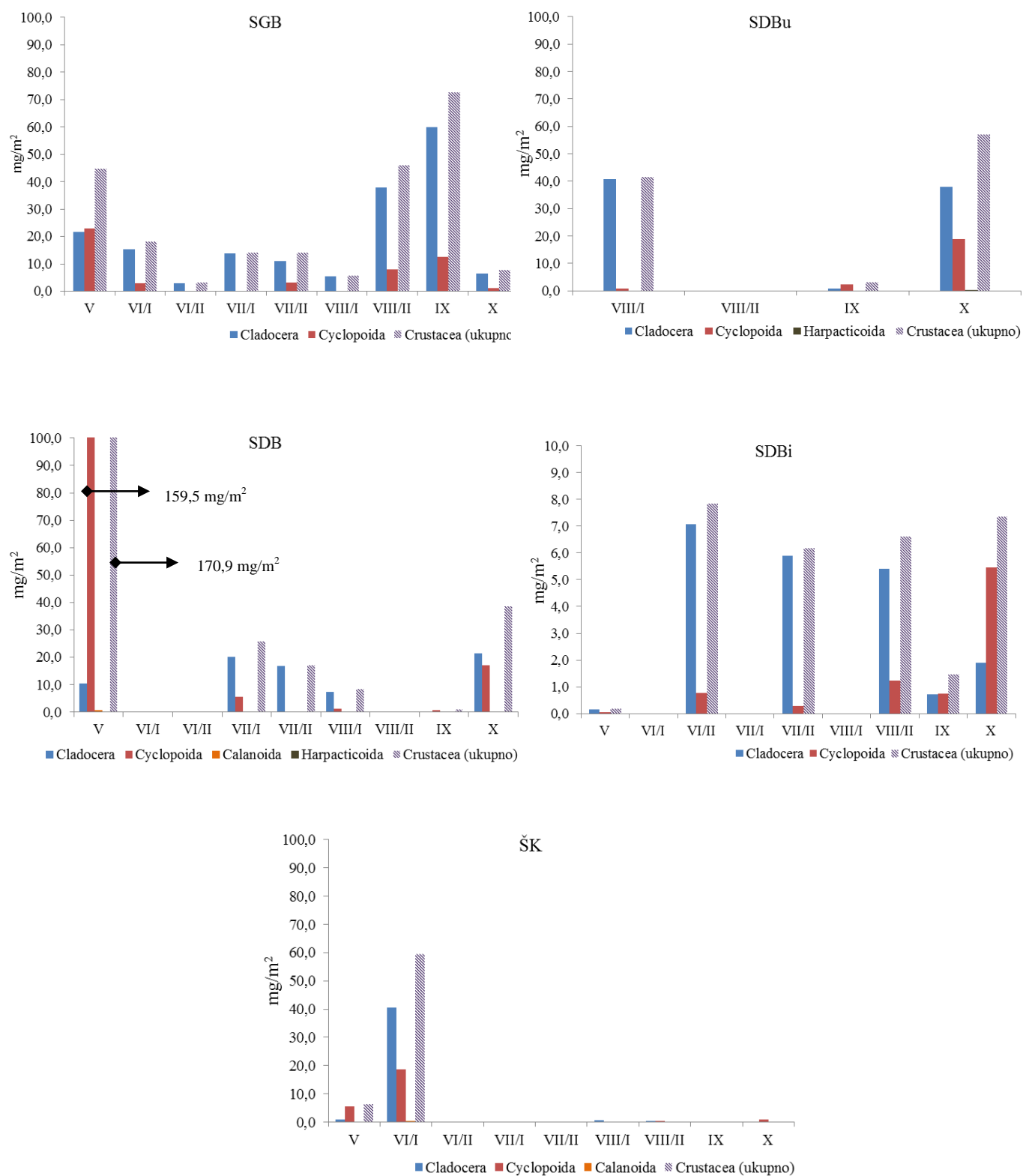
Slika 11 Vremenske promjene biomase ( \text{mg}/\text{m}^2 ) planktonskih rakova u sedimentu litorala postaje sa submerznim makrofitima (SGB), bez makrofita (SDBu, SDB, SDBi) i postaje s flotantnim makrofitima (ŠK).
