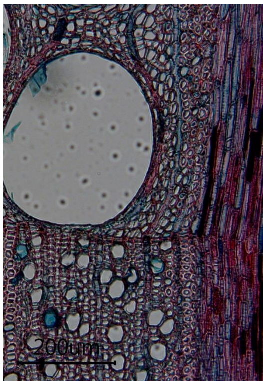
Slika 115. Poprečni presjek drva hrasta, povećanje objektiva 10X
