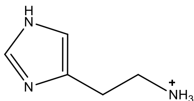
Slika 14: Strukturna formula histamina (a) i analoga gvanidina (b) pri fiziološkom pH ( \sim 7,4 )
