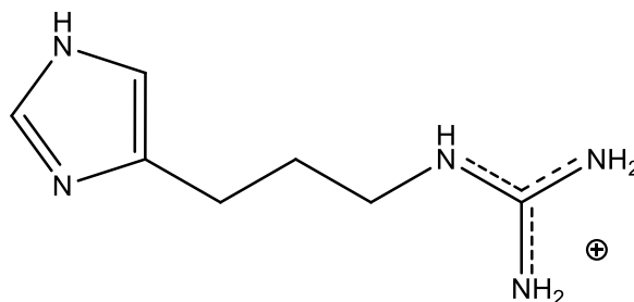
Slika 14: Strukturna formula histamina (a) i analoga gvanidina (b) pri fiziološkom pH ( \sim 7,4 )
