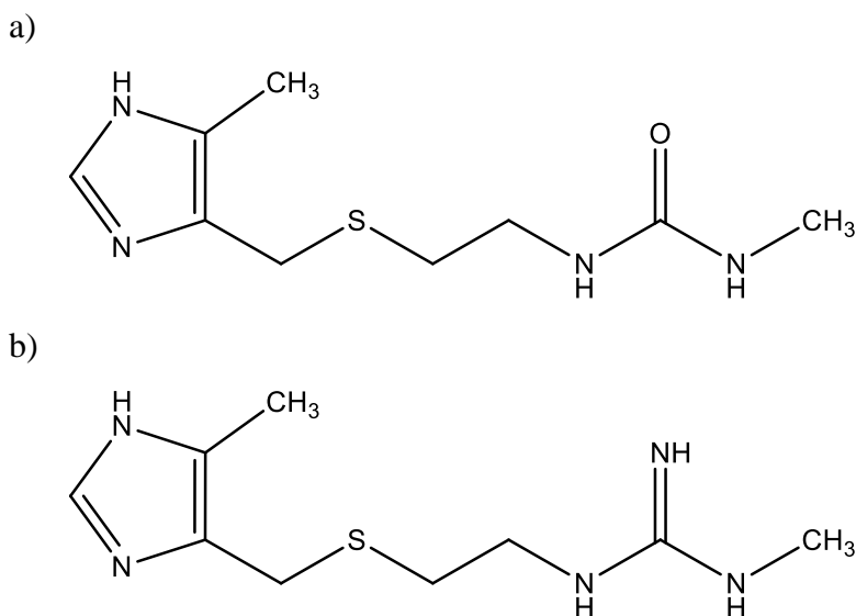
Slika 19: Strukturne formule analoga metiamida: a) urein analog i b) analog gvanidina
