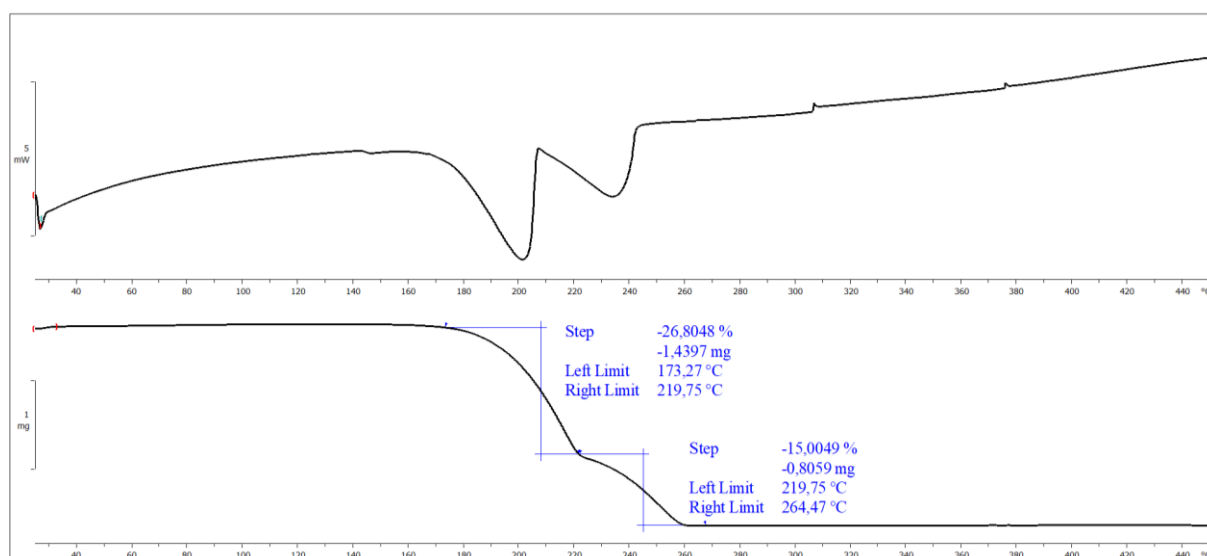
Slika D7. DSC i TGA krivulja spoja A2
