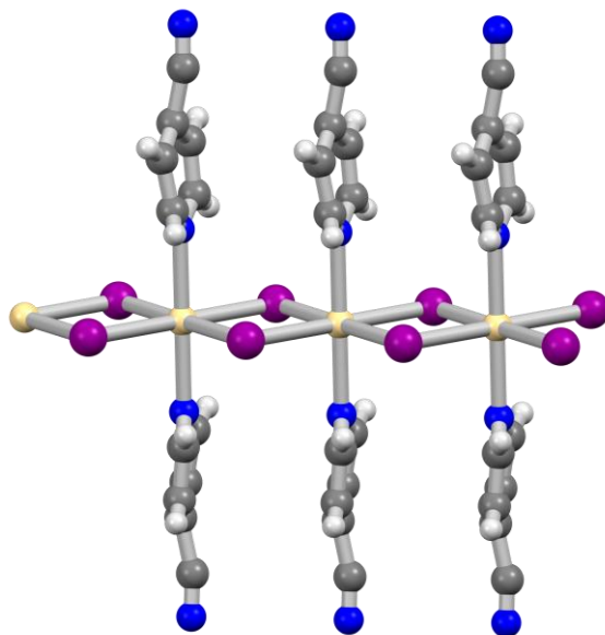
Slika 8. Struktura [CdI_2(4-CNpy)_2]_n 30
