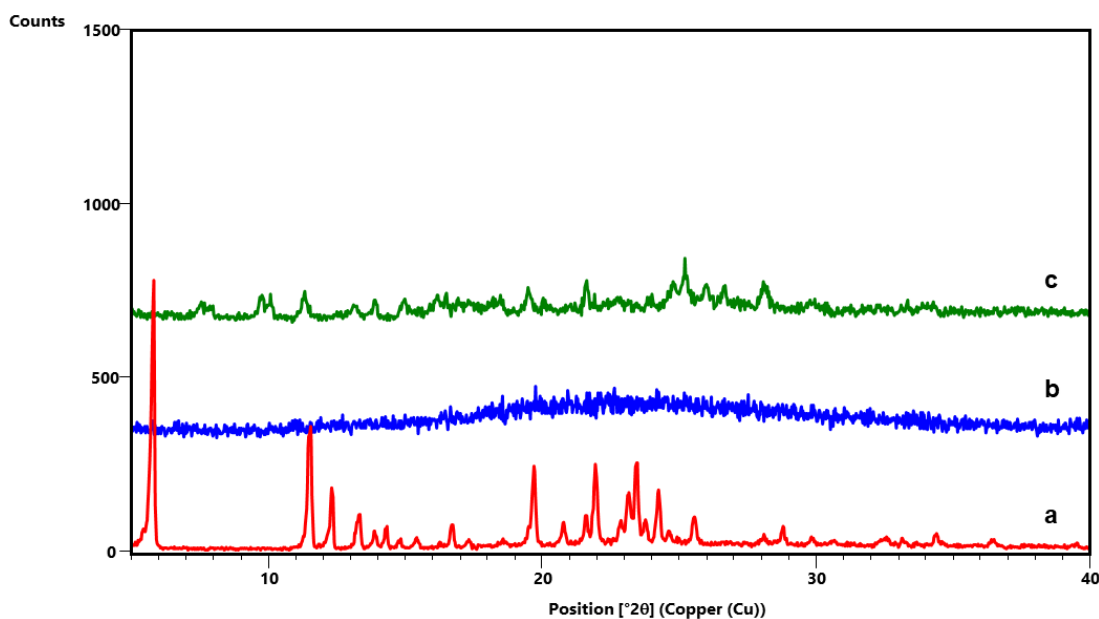
Slika D10. Difraktogrami: a) dpz , b) produkta dobivenog mljevenjem reakcijske smjese dpz i ipfb u stehiometrijskom omjeru 1:1, c) produkta dobivenog mljevenjem reakcijske smjese dpz i ipfb u stehiometrijskom omjeru 1:2
