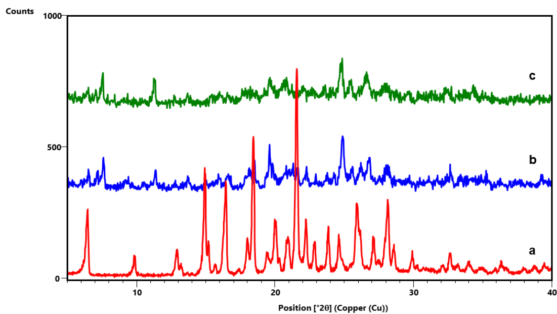
Slika D12. Difraktogrami: a) dpzHCl , b) produkta dobivenog mljevenjem reakcijske smjese dpzHCl i 13tfib u stehiometrijskom omjeru 1:1, c) produkta dobivenog mljevenjem reakcijske smjese dpzHCl i 13tfib u stehiometrijskom omjeru 1:2
