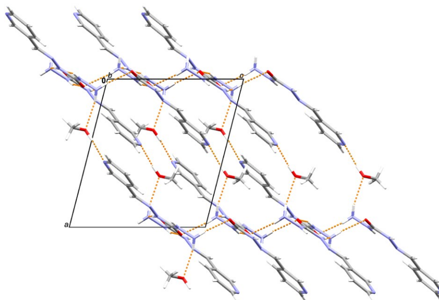
Slika XXXII. Prikaz pakiranja molekula s istaknutim vodikovim vezama, u kristalnoj strukturi \text{H}_2\text{L}^{3\text{py}} \cdot \text{MeOH} duž kristalografske b -osi gdje su vodikove veze N–H \cdots O i O–H \cdots N tipa označene isprekidanim narančastim linijama
