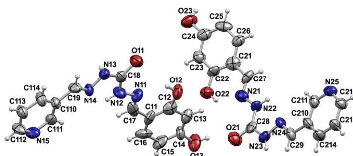
Slika 28. Molekulska struktura H_3L^{3py-4OH} , simetričnu jedinku čine 2 molekule H_3L^{3py-4OH} . Elipsoidi pomaka nevodikovih atoma prikazani su s vjerojatnošću od 50 %, a vodikovi su atomi prikazani kao kuglice proizvoljnog radijusa.
