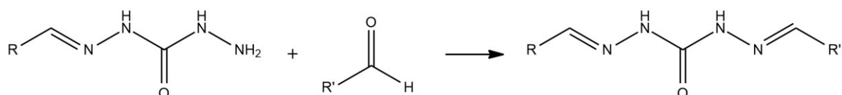
Shema 3. Postupak priprave a) monosupstituiranih karbonohidrazida i b) drugi korak u sintezi disupstituiranih karbonohidrazida
