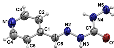
Slika 18. Molekulska struktura H_2L^{4py} . Elipsoidi pomaka nevodikovih atoma prikazani su s vjerojatnošću od 50 %, a vodikovi su atomi prikazani kao kuglice proizvoljnog radijusa
