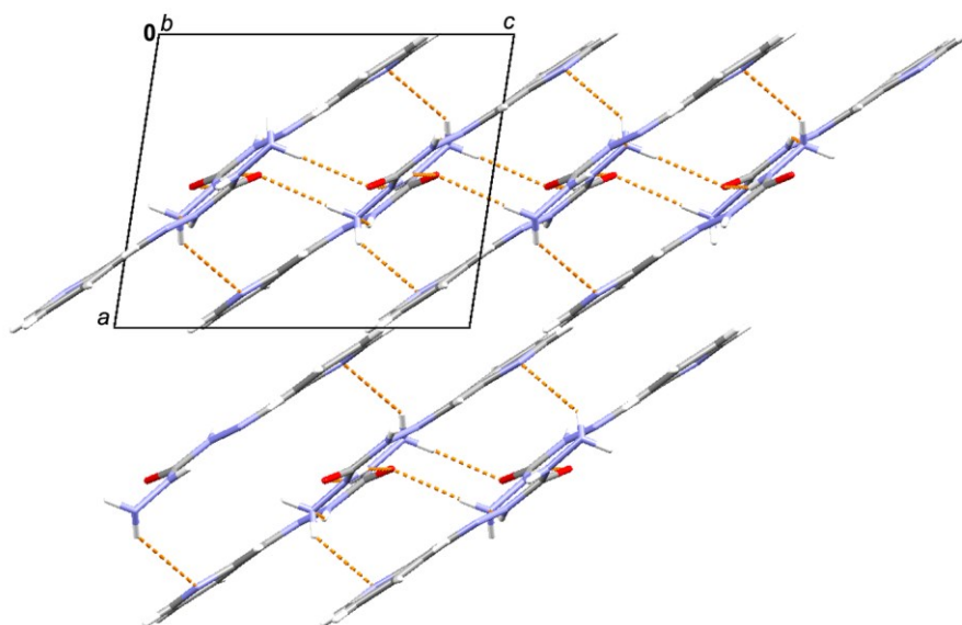
Slika XXXI. Prikaz pakiranja molekula s istaknutim vodikovim vezama, u kristalnoj strukturi \text{H}_2\text{L}^{2\text{py}} duž kristalografske b -osi gdje su vodikove veze N–H \cdots O i N–H \cdots N tipa označene isprekidanim narančastim linijama
