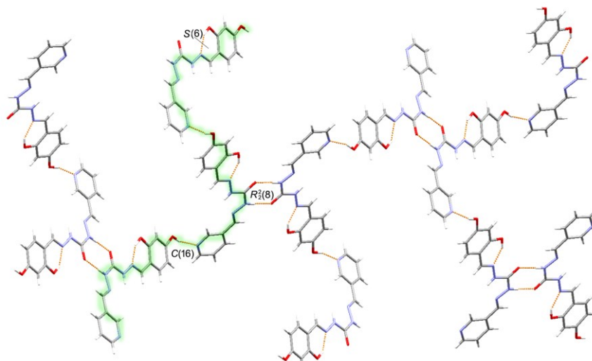
Slika 27. Prikaz pakiranja molekula, s istaknutim graf-set motivima vodikovih veza, u strukturi H_3L^{3py-4OH} \cdot 0,5(MeOH) , duž kristalografske a -osi
