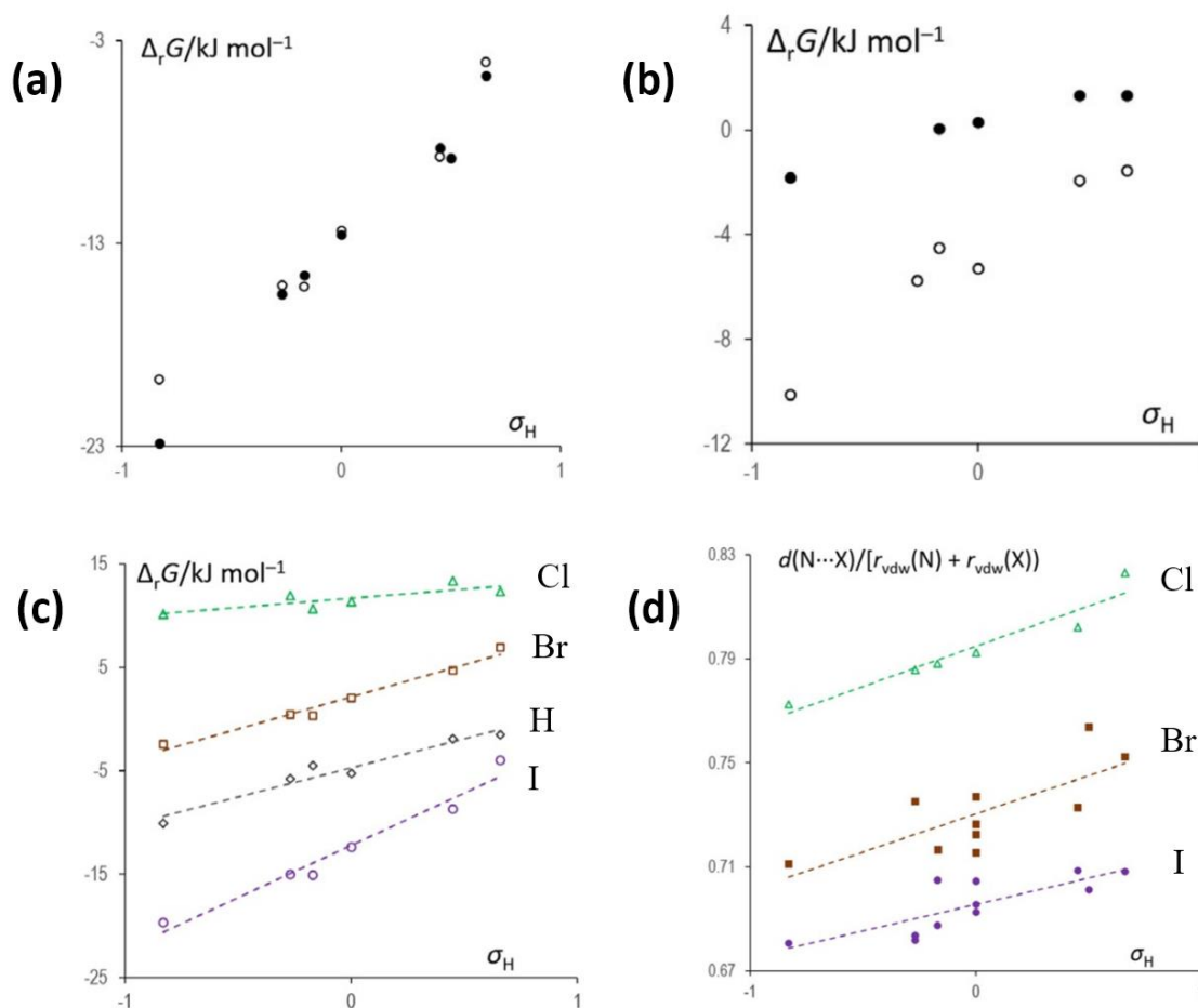
Slika 24. Prikaz ovisnosti reakcijske Gibbsove energije nastajanja kompleksa para -supstituiranog piridina i (a) N -jodsukcinimida u acetonitrilnoj otopini (puni krugovi) i plinu (računom; kružnice), (b) sukcinimida u acetonitrilnoj otopini (puni krugovi) i plinu (računom; kružnice) te (c) N -halogensukcinimida i sukcinimida u plinu (računom) o Hammettovoj konstanti supstituenta. (d) Omjer duljine interakcije i sume van der Waalsovih radijusa interagirajućih atoma u ovisnosti o Hammettovoj konstanti (udaljenosti za brom i jod su dobivene iz difrakcijskih eksperimenata, a za klor računom). Uzimajući u obzir da Hammetova konstanta para -supstituenata ovisi linearno o pK_a vrijednosti odgovarajućeg piridina, 92,93 a pK_a vrijednost o logaritmu konstante stabilnosti kompleksa, 94 iz usporedbe veličina dobivenih eksperimentom i Hammetovih konstanti mogu se izvoditi zaključci o prirodi spomenutih interakcija: ukoliko prate jednake trendove, može se reći da je priroda interakcija slična. Preuzeto s ref. 90.
