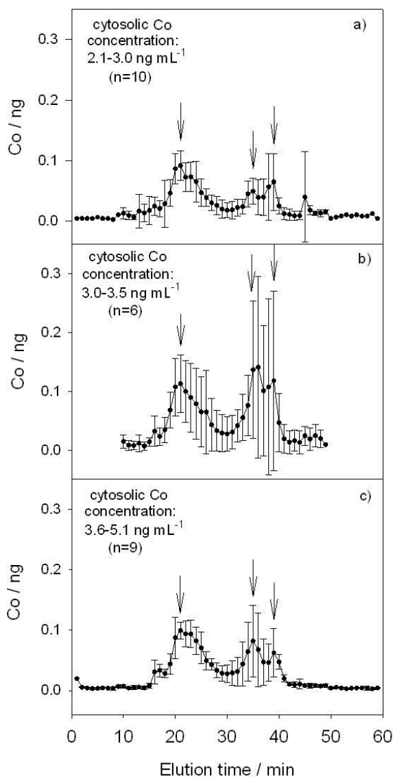
Slika 1. Raspodjele Co među biomolekulama različitih molekulskih masa u citosolima jetara klenova ( S. cephalus ) dobivene SEC-HPLC razdvajanjem na koloni Superdex™ 200 10/300 GL i mjerenjem na HR ICP-MS-u. Analizirani uzorci su podijeljeni u tri skupine, prema citosolskim koncentracijama Co ( \text{ng mL}^{-1} ) u jetrima klenova. Oznaka slike u radu ESI I .
