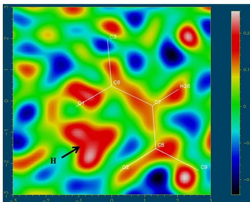
Slika 50. Razlikovna mapa elektronske gustoće karbonilne odnosno hidroksilne skupine jedne od molekule b4pm -a prisutne u formulskoj jedinici kokristala (b4pm)(1,3-tfib) s naznačenim položajem atoma vodika između atoma O1 i O2 . Visina i širina slike iznose 6 Å, a elektronska gustoća izražena je u e/\text{Å}^2 .
