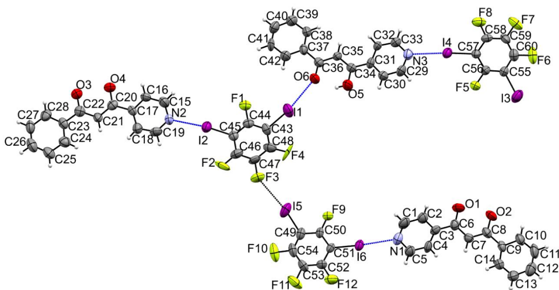
Slika 29. ORTEP prikaz molekula u strukturi kokristala (b4pm)(1,3-tfib) s označenim atomima, halogenskom vezom (plavo) te interhalogenim kontaktom (crno). Elipsoidi pomaka za nevodikove atome prikazani su na razini vjerojatnosti od 50 %. Vodikovi atomi prikazani su sferama radijusa 0,15 Å
