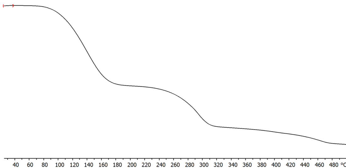
Slika D24. TG krivulja kokristala (b4pm)(ipfb)
