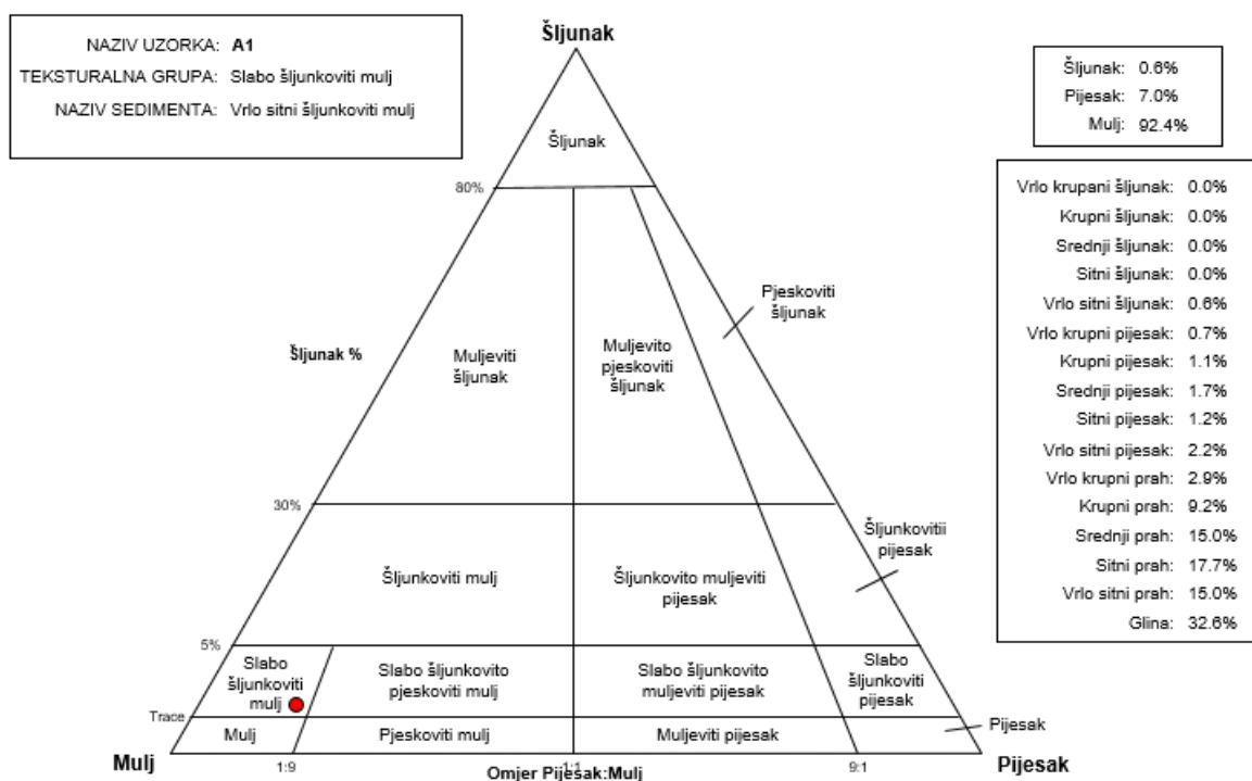
Slika 10. Granulometrijski sastav sedimenata iz uzorka A1 u trokomponentnom dijagramu šljunka, pijeska i mulja prema Folku (1954).
