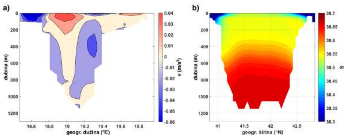
Slika 31. Vertikalni presjeci (a) morskih struja u Otrantskim vratima (40 ^{\circ}\text{N} , pozitivne vrijednosti označavaju struju prema sjeveru), i (b) saliniteta na poprečnom transektu u južnom Jadranu na 17.5 ^{\circ}\text{E} geografske dužine, usrednjenih u razdoblju 1980. - 2012., za simulaciju MED12F3.
