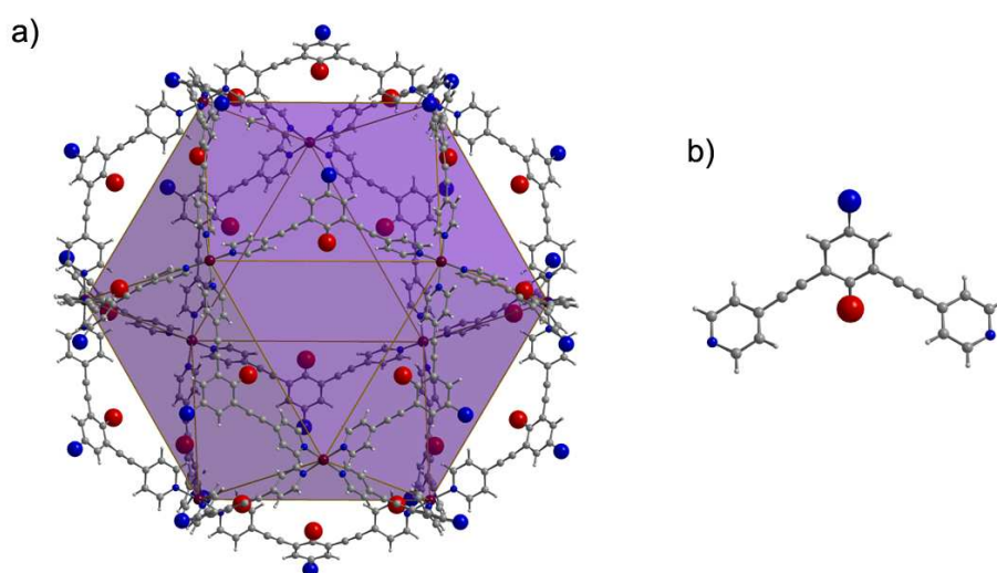
Slika 16. a) Struktura „metaloorganskog kuboktaedra“ [\text{Pd}_{12}(\text{L})_{24}]^{24+} ; b) pojednostavljeni prikaz poveznice L koja pripada skupini 2,6-bis((2-piridin-4-il)etil)fenil liganada (supstituenti na položaju 2 i 4 središnjeg benzenskog prstena su istaknuti kao plave, odnosno crvene kuglice većeg promjera). Shema boja: Pd-ljubičasto, C-sivo, N-plavo, O-crveno i H-bijelo. 12
