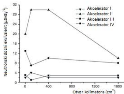
Slika 28. Neutronska dozna ekvivalent u \mu\text{Sv} po 1 Gy fotonske doze u izocentru za sva četiri akceleratora u točki C. Kut kućišta je 0^\circ . Veličine snopova prikazane su u \text{cm}^2 [8].
