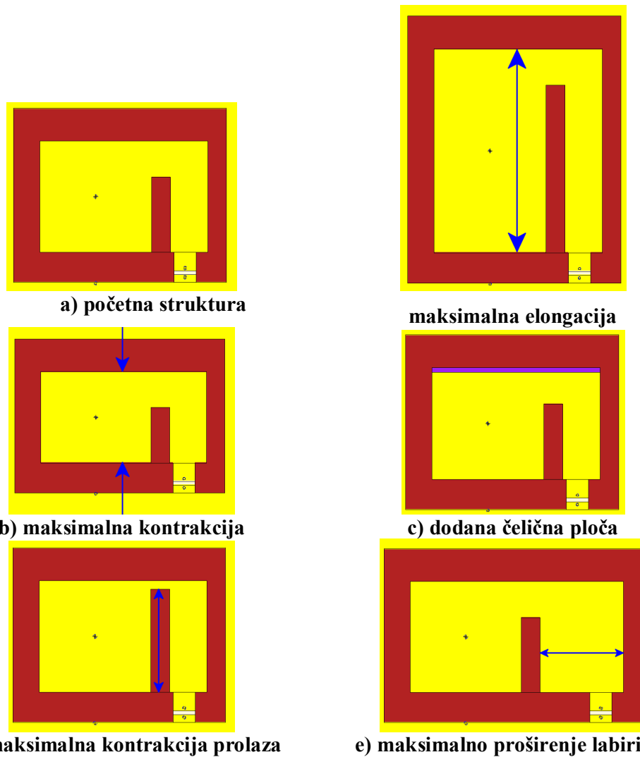
Slika 27. Tlocrti bunkera u istraženim slučajevima. Beton je označen crvenom bojom, zrak žutom, a čelična ploča ljubičastom.
