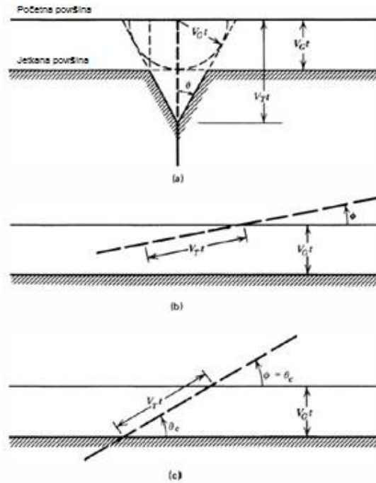
Slika 11. Model jetkanja: (a) kad je latentni trag okomit na površinu detektora, (b) kad je latentni trag pod kutom \phi < \theta_c i (c) kad je latentni trag pod kritičnim kutom \theta_c [26].
