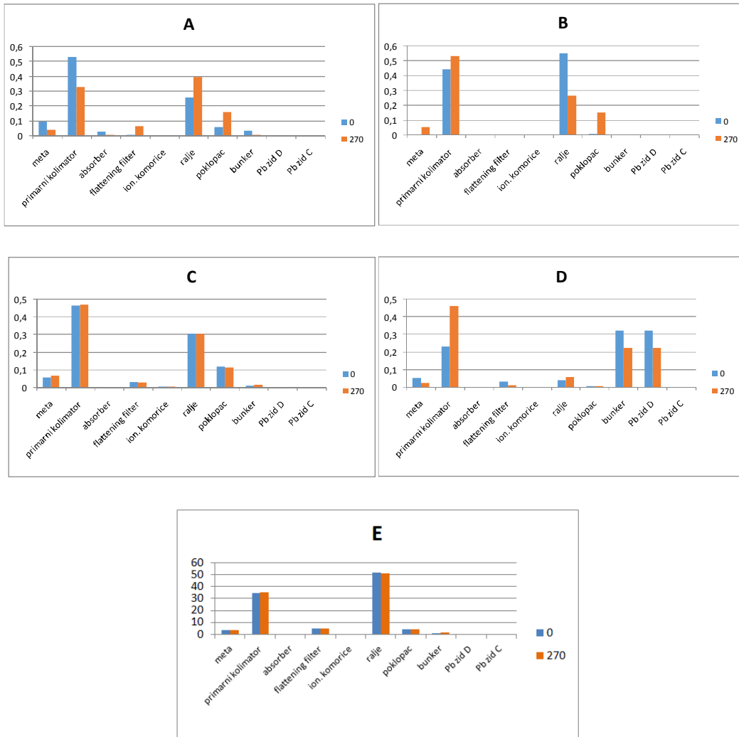
Slika 35. Prikaz neutronskeg toka prema mjestu nastanka neutrona za mjerne položaje A, B, C, D i E.
