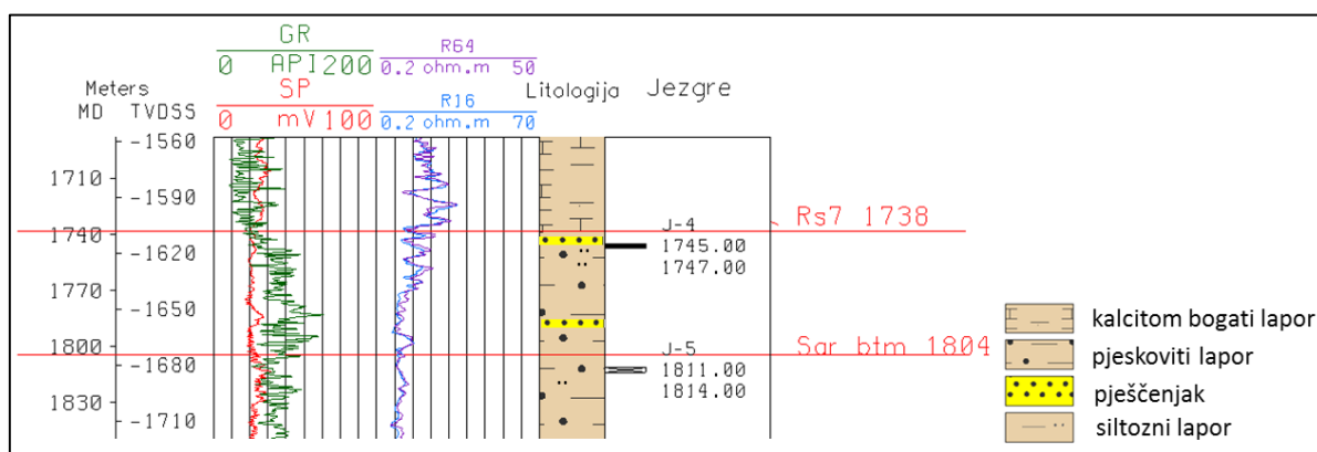
Slika 7.12. Karotažni i litološki podatci iz bušotine B-1 (istraživani interval)
