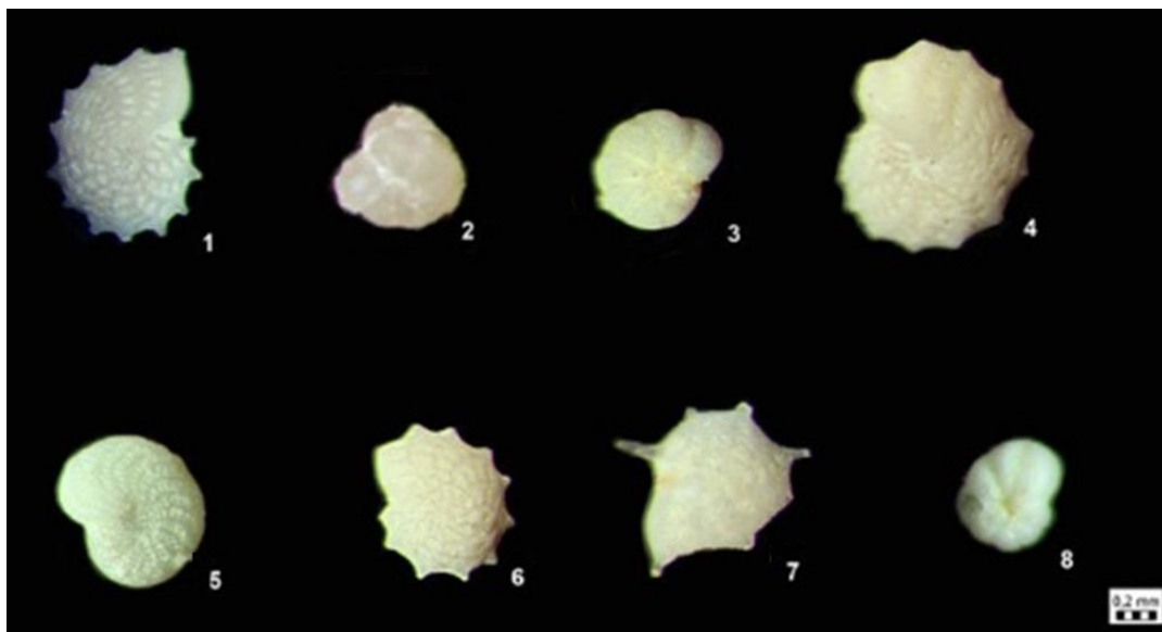
Slika 7.3. Značajne vrste foraminifere izdanka 5: 1- Elphidium josephinum , 2- Anomalinoides dividens , 3- Porosononion granosum , 4- Elphidium aculeatum , 5- E. hauerinum , 6- E. reginum , 7- E. reginum , 8- Nonion bogdanowitzi
