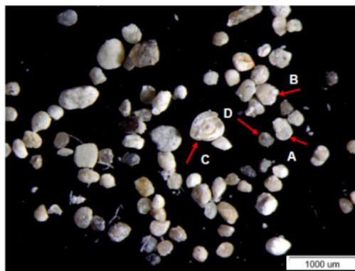
Slika 5.9. Bušotina B-12, interval 2220-2230 m, zajednica bentičkih foraminifera sarmata, A- Anomalinoidea dividens , B- Cibicides sp., C- Miliolida , D- Nonion sp. (Veseli et al., 2014)
