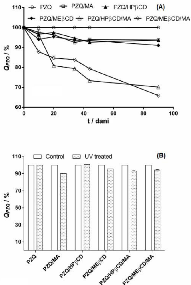
Slika 44. Promjene u koncentraciji PZQ-a u odabranim uzorcima tijekom ispitivanja kemijske stabilnosti lijeka metodom ubranog starenja na 40 \pm 2 \text{ }^\circ\text{C} / 75 \pm 5\% \text{ RH} (A) te tijekom ispitivanja fotostabilnosti (B).
