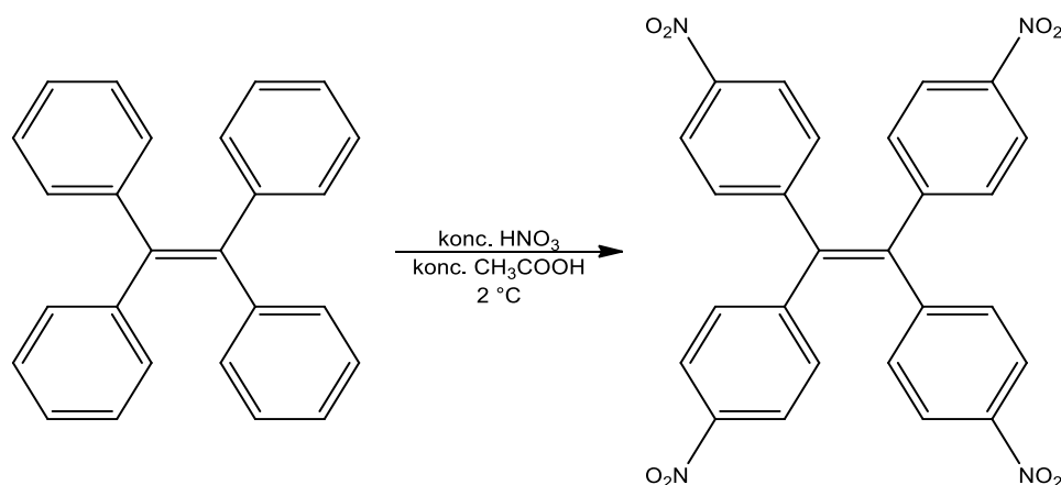
Slika 32. Sinteza aromatskog tetranitro spoja (1)
