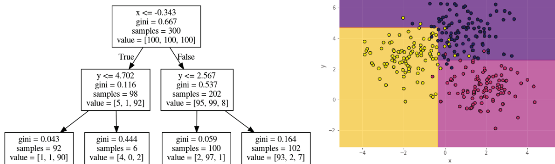
Slika 3.6: Stablo odlučivanja dubine 2 (lijevo) i klasifikacija točaka na temelju tog stabla (desno).
