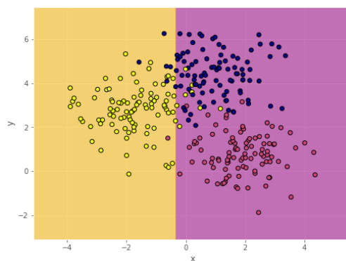
Slika 3.5: Stablo odlučivanja dubine 1 (lijevo) i klasifikacija točaka na temelju tog stabla (desno).
