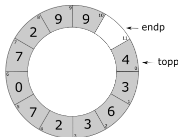
Slika 2.15: Cirkularno polje
