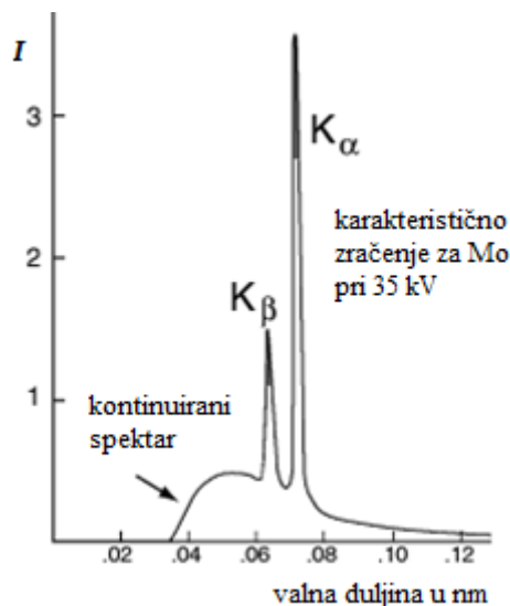
Slika 3. Spektar zračenja
