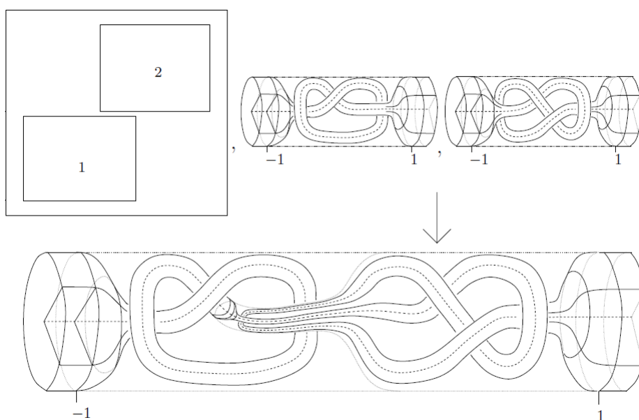
Slika 3.5: Primjer djelomičnog preklapanja domena u definiciji 3.1.8, [3]
