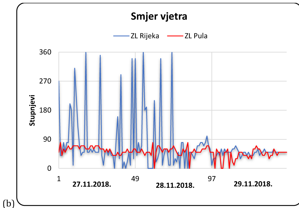
Slika 36. Prikaz (a) brzine vjetra (u čvorovima) i (b) smjera vjetra za Zračnu luku Rijeka i Zračna luka Pula od 27. do 29. studenoga 2018. 48 mjerenja u jednom danu (svakih pola sata), ukupno 144 mjerenja u 3 dana. 1 čvor = 0,5144 m/s.
