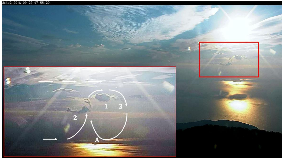
Slika 34. Obrabljena fotografija koja prikazuje nebo iznad Zračne luke Rijeka u terminu 7:55 UTC, 29. rujna 2018. 1 – kumulusa (Cu), 2 – manji fragmentirani Cu koji će se stopiti s većim, 3- mali oblačići koji se otkidaju od Cu i nestaju, A – mjerna postaja. Strelice prikazuju strujanje zraka.
