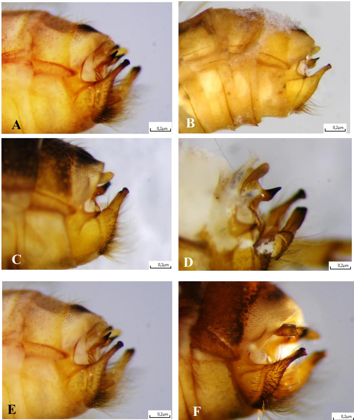
Slika 37. A-F. Lateralni izgled muškog genitalnog aparata vrsta roda Potamophylax : A - P. latipennis , TPLAT_2, B - lateralni izgled P. cingulatus , TPCIN_1, C – P. latipennis primjerak TPLAT_3, rijeka Zrmanja, izvor, D - P. latipennis , primjerak TPLAT_4, rijeka Rječina, izvor, E - P. latipennis , primjerak TPLAT_1, rijeka Una, Srb, F - P. latipennis , primjerak TPLAT_7, rijeka Gacka, izvor Tonkovića vrilo (Foto: Mladen Kučinić).
