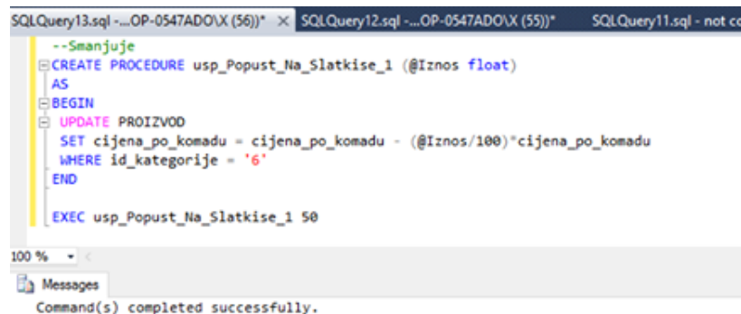
Slika 3.15: Kreiranje procedure
