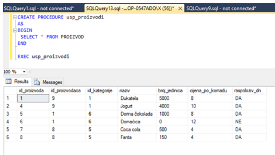
Slika 3.14: Kreiranje procedure
