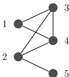
Slika 2.1: Nebipartitan graf
