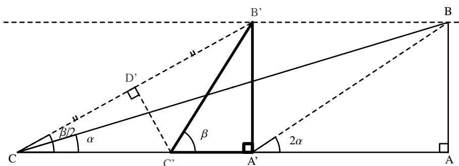
Slika 2.4: Novi trokut A'B'C' s kutom \beta
