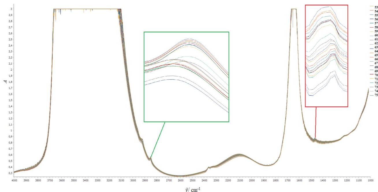
Slika 14. FT-IR spektri DPPE-a u temperaturnom intervalu od 53 °C do 75 °C tijekom prvog mjerenja (R1), s uvećanim vrpčama simetričnog istežanja \nu_s\text{CH}_2 i strižne deformacije metilenske skupine \gamma\text{CH}_2 .
