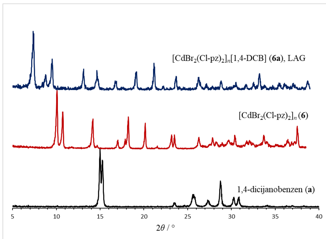
Slika D16. Usporedba difraktograma polikristalnih uzoraka reaktanata [\text{CdBr}_2(\text{Cl-pz})_2]_n (6) i 1,4-dicijanoobenzenu (a) i produkta mljevenja potpomognutog kapljevinom (6a).
