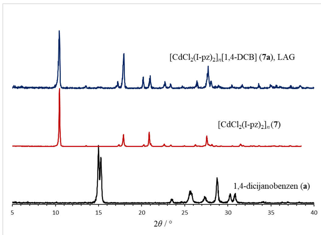
Slika D17. Usporedba difraktograma polikristalnih uzoraka reaktanata [\text{CdCl}_2(\text{I-pz})_2]_n (7) i 1,4-dicijanoobenzenu (a) i produkta mljevenja potpomognutog kapljevinom (7a).
