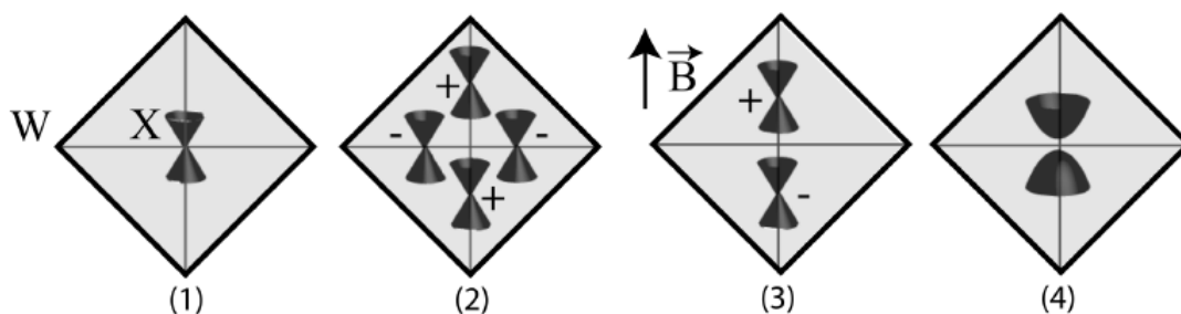
Slika 2.5: (1) Stanja u Diracovoj točki su četverostruko degenerirana. (2) Pojavljuju se četiri Weylove točke lomljenjem simetrije na prostornu inverziju. Kiralnost točaka označena je predznacima + i -. (3) Pojavljuju se dvije Weylove točke zbog lomljenja vremenske simetrije primjenom magnetskog polja u smjeru takvom da kristalna simetrija ostane sačuvana. (4) Primjena magnetskog polja u bilo kojem drugom smjeru lomi rotacijsku simetriju i dolazi do izolatorskog stanja.
