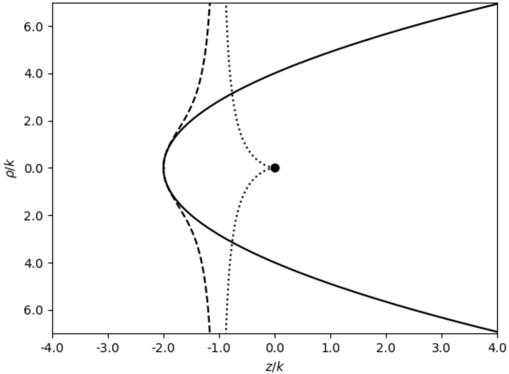
Slika 3.3: Sjenu Rutherfordovog raspršenja crtana je punom crtom. Krivulja koju čine točke najbližeg približenja nacrtana je crtkano, a nefizikalni dio te krivulje točkasto.
