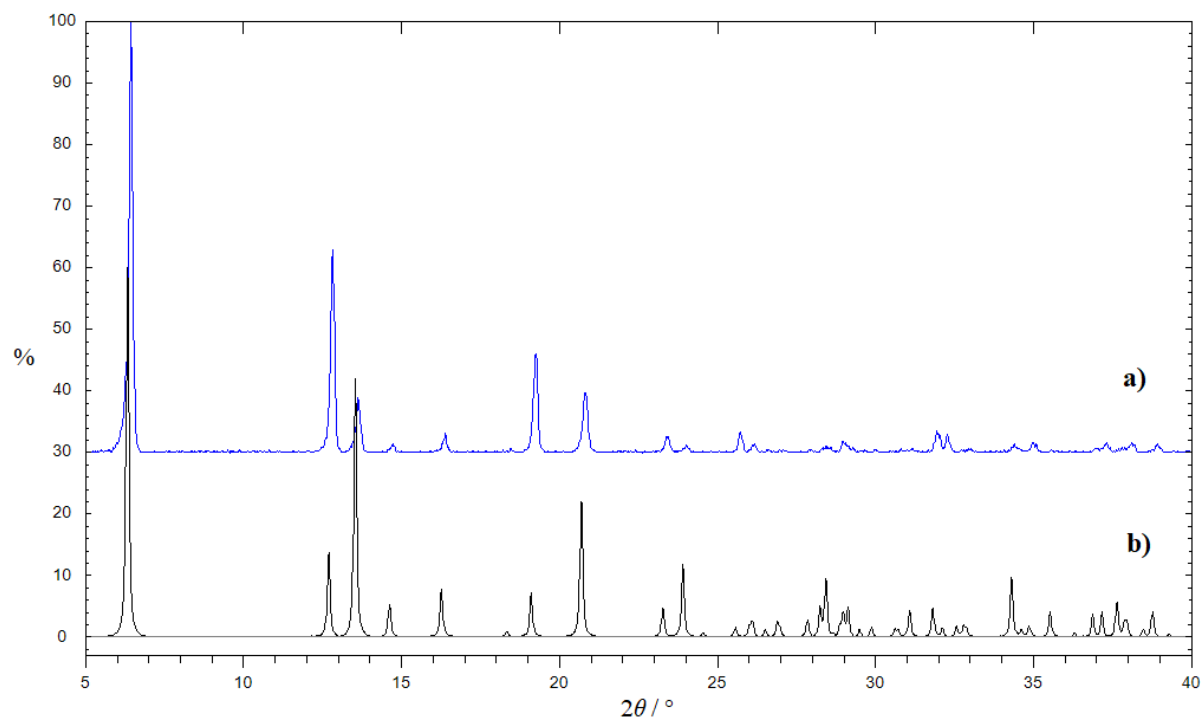
Slika D1. Difraktogrami prahova spoja [\text{CdCl}_2(3\text{-NO}_2\text{py})_2]_n (1): a) otopinska sinteza (plavo), b) izračunati difraktogram praha (crno).
