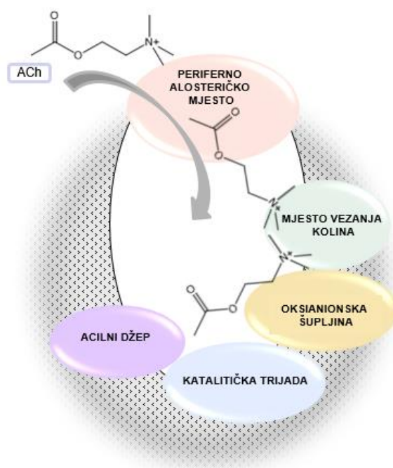
Slika 2. Shematski prikaz aktivnog mjesta kolinesteraza s naznačenim strukturnim domenama i supstratom acetilkolinom (ACh). Strelica označava smjer ulaska i pozicioniranja acetilkolina u aktivno mjesto kolinesteraza. (preuzeto i prilagođeno prema ref. 8)
