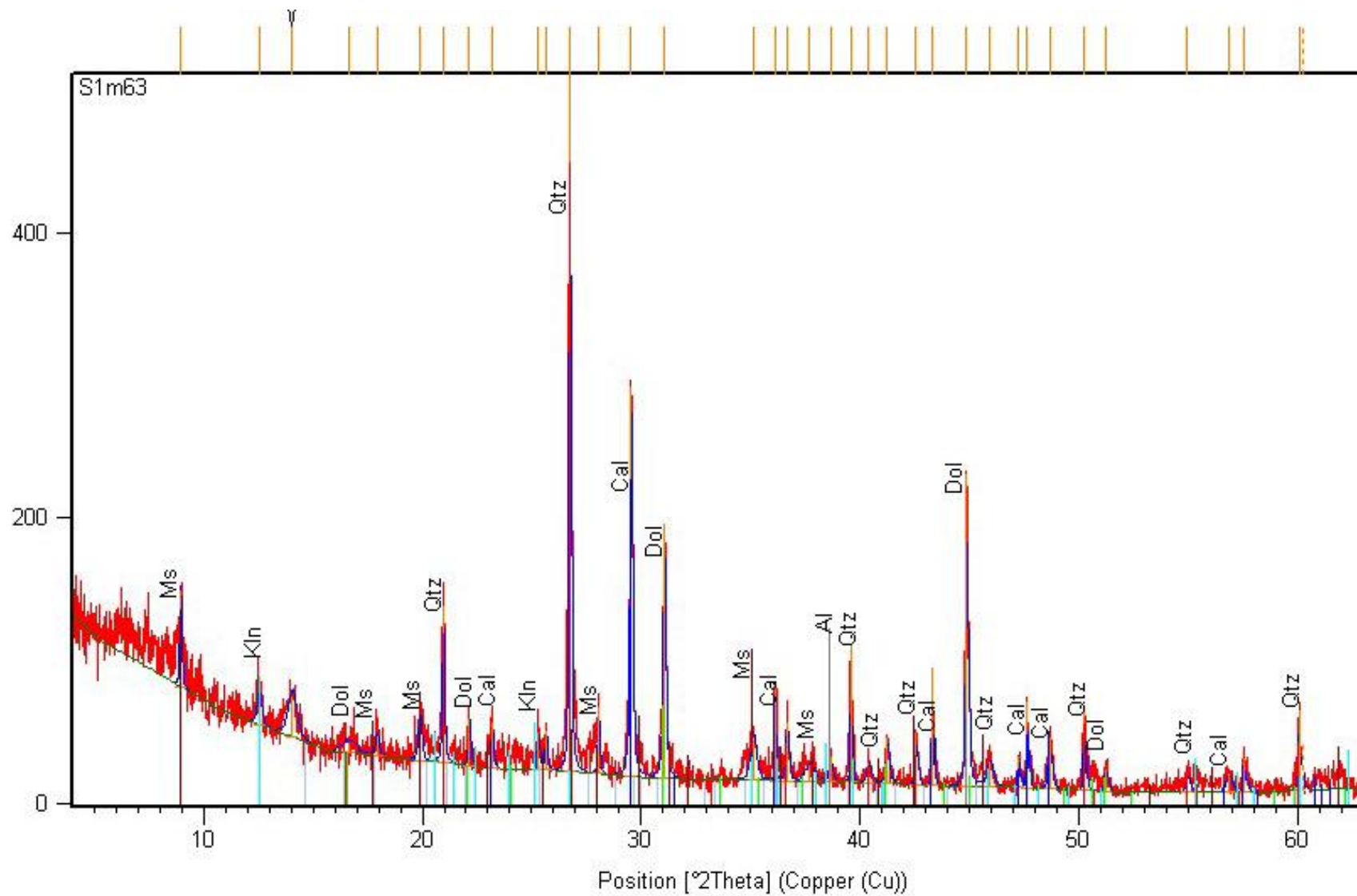
Prilog24. Rendgenogram uzorka SF, točka A
