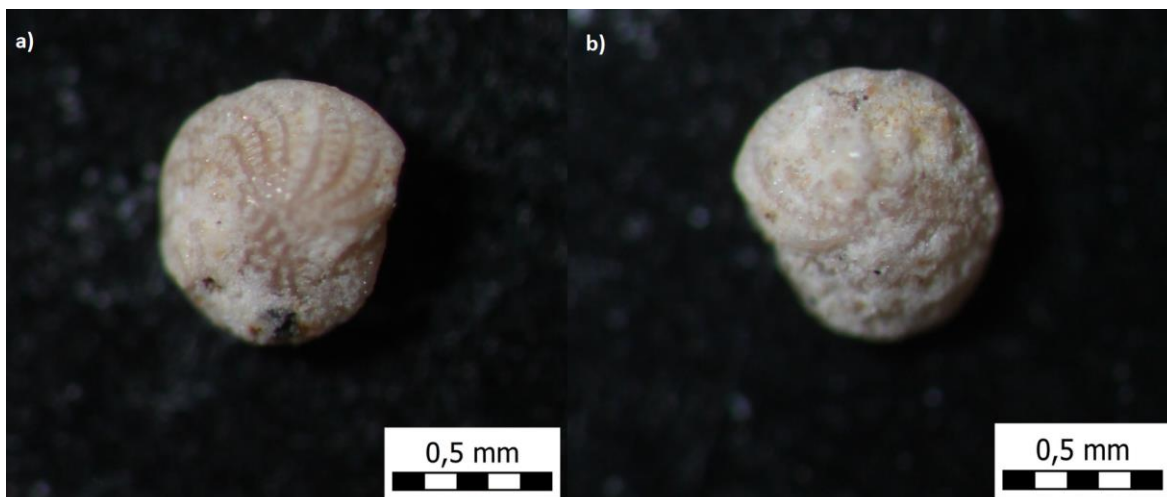
Slika 19. a), b) Elphidium crispum , uzorak B, frakcija 250 \mu\text{m}
