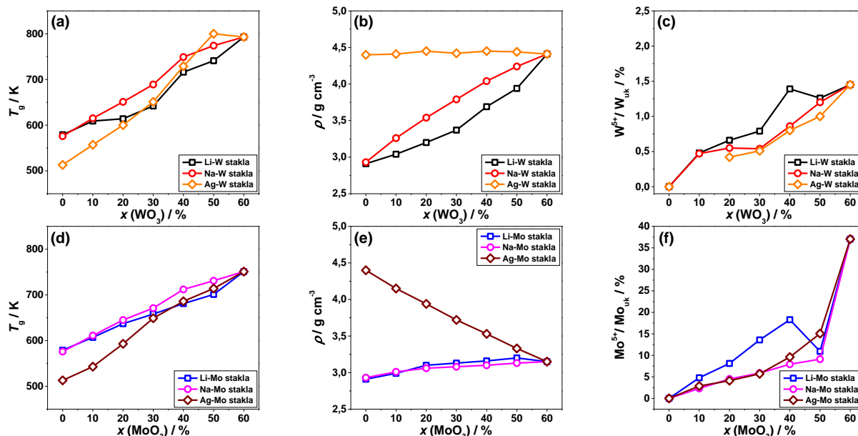
Slika 20. Ovisnost vrijednosti temperature staklišta, T_g , (a i d); gustoće, \rho , (b i e); i omjera W^{5+}/W_{\text{uk}} odnosno Mo^{5+}/Mo_{\text{uk}} (c i f) o množinskom udjelu WO_3 i MoO_3 za sva istraživana stakla.
