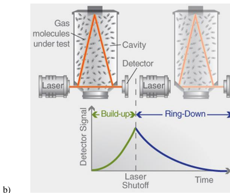
Slika 23. a) Laserski spektrometar L2130i tvrtke Picarro ; b) princip mjerenja
